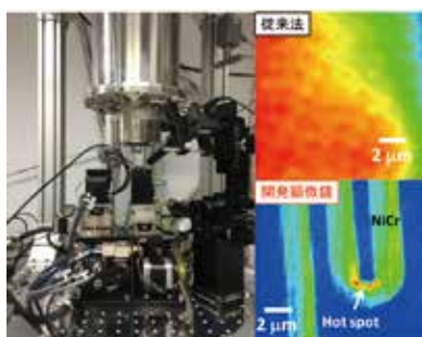
THz近接場顕微鏡と電流分布のナノスケール可視化
