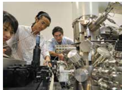
超高真空電子顕微鏡下でAFMを用いた力学計測と元素同定
